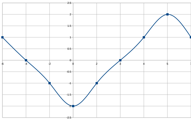
Courbe de f
