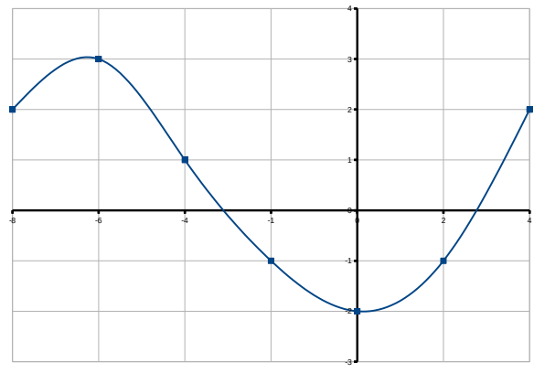
Courbe de g(x)
