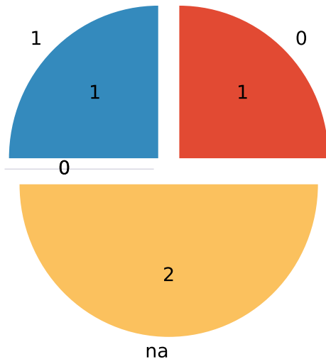
Rai (total=4)
