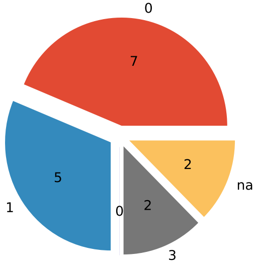
Cal (total=16)
