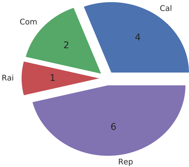
len (total=13)
