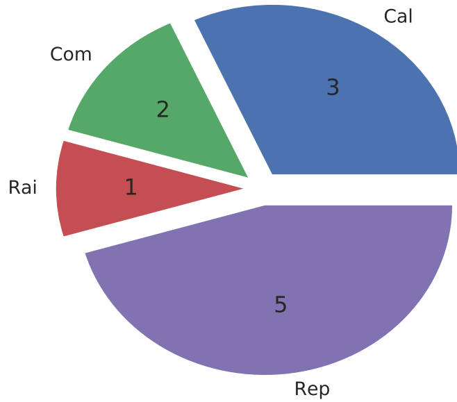
sum (total=11.0)
