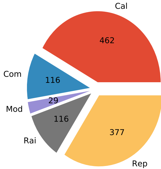
len (total=1100)
