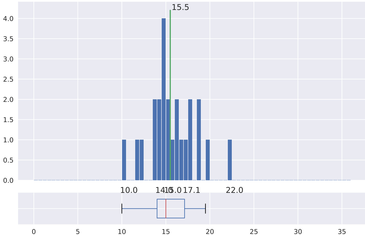
Histogramme pour Bbmai
