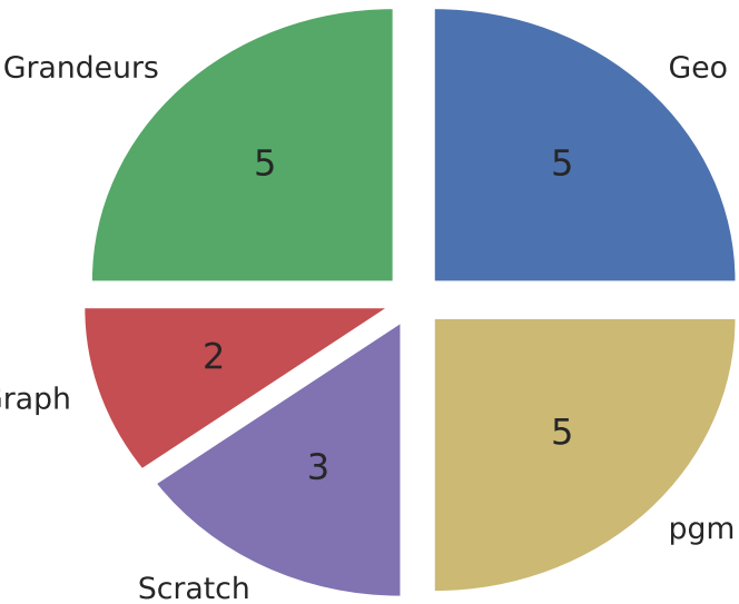
len (total=20)
