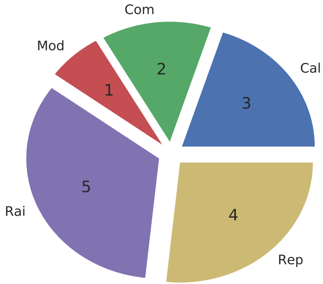
len (total=15)
