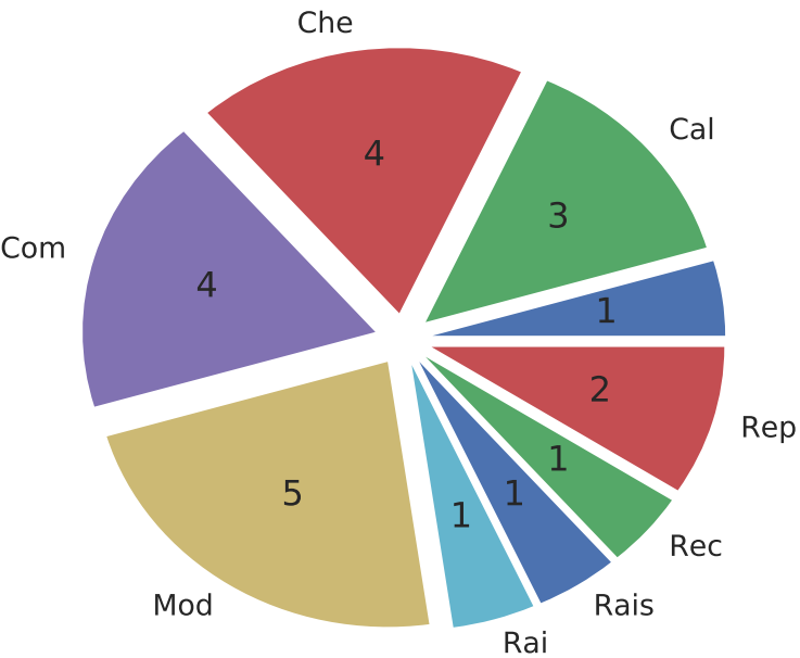
len (total=22)
