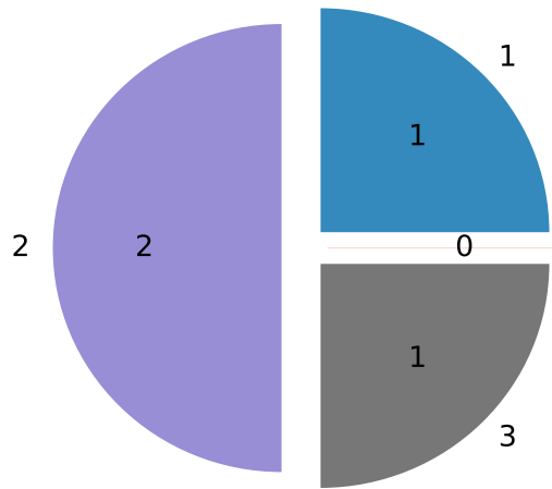
4op (total=4)
