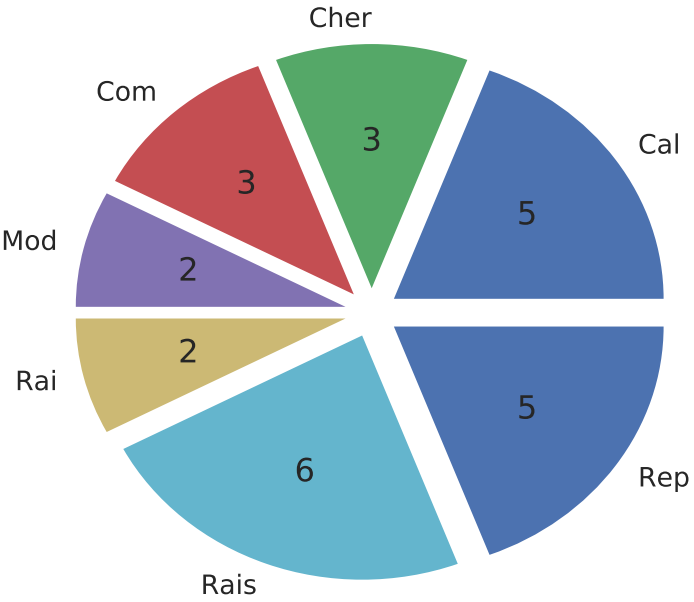
len (total=26)
