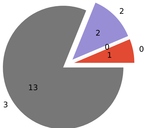
Cal (total=16)
