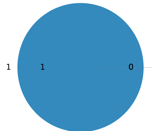
Mod (total=1)
