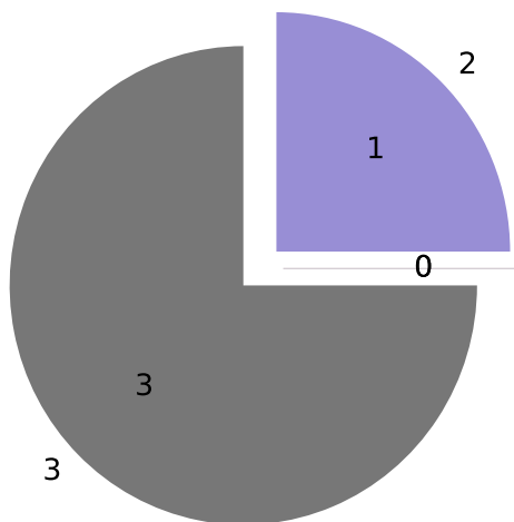
Rai (total=4)
