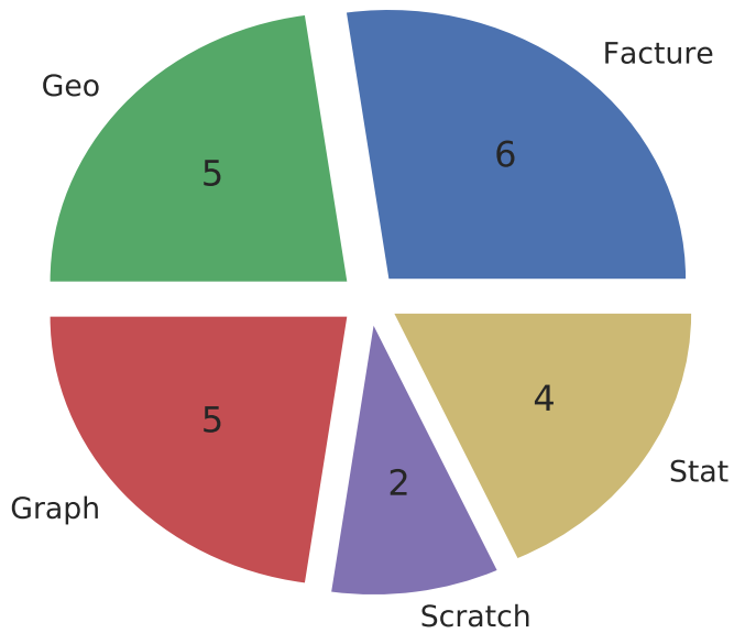
len (total=22)
