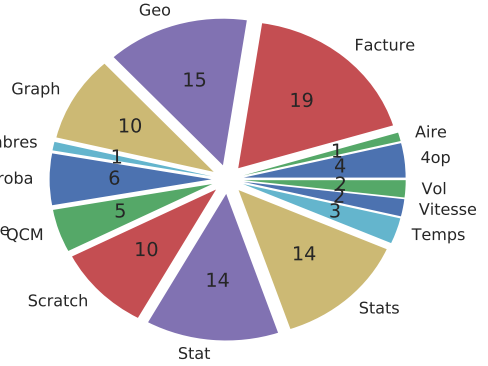
sum (total=106)
