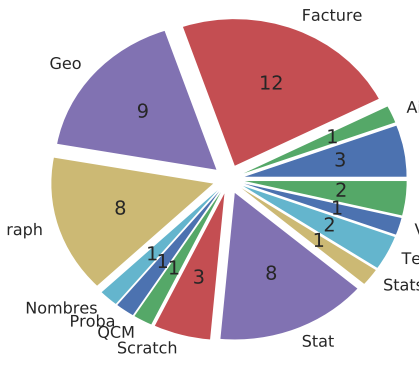
len (total=53)
