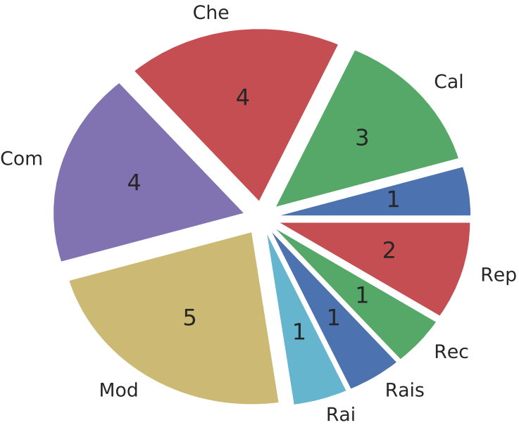
len (total=22)
