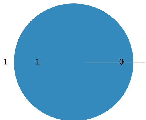
Sym (total=1)
