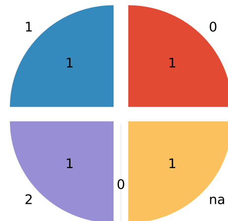
Prop (total=4)
