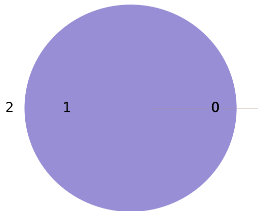
Frac (total=1)
