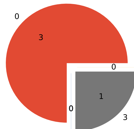
pgm (total=4)
