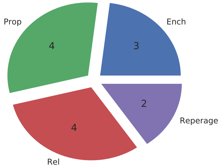
len (total=13)
